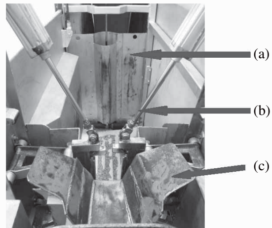
Figura 1. Vista del interior del cajón de noqueo, mostrando la puerta de ingreso tipo guillotina (a), el dispositivo de sujeción cervical (b) y el eleva mentón (c).
