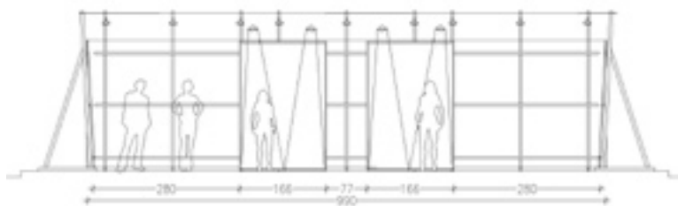
Elevación interior
