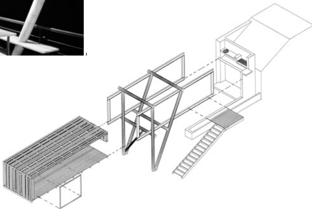
Axonométrica de elementos: Fundación, estructura de rollizos y envoltivo de tablas
