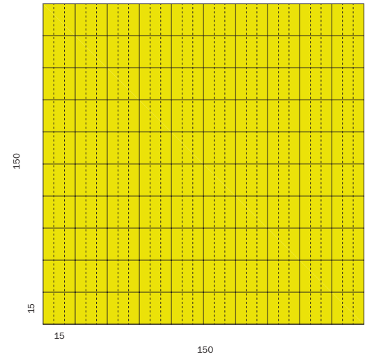
Plantas de membrana textil, cien piezas de 4,5 m x 4,5 m E. 1: 750
