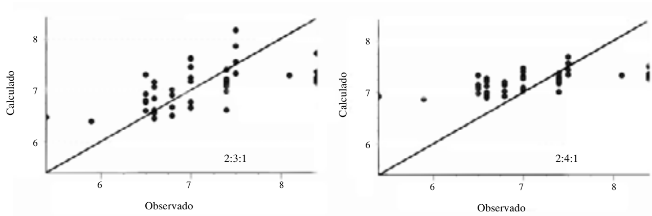
Figura 4. Valores observados en función del valor calculado. Actual values in relationship with calculate value.
