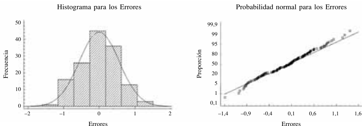
Figura 3. Histograma de frecuencias y gráfico de probabilidad normal. Frequency histogram and normal probability plot.
