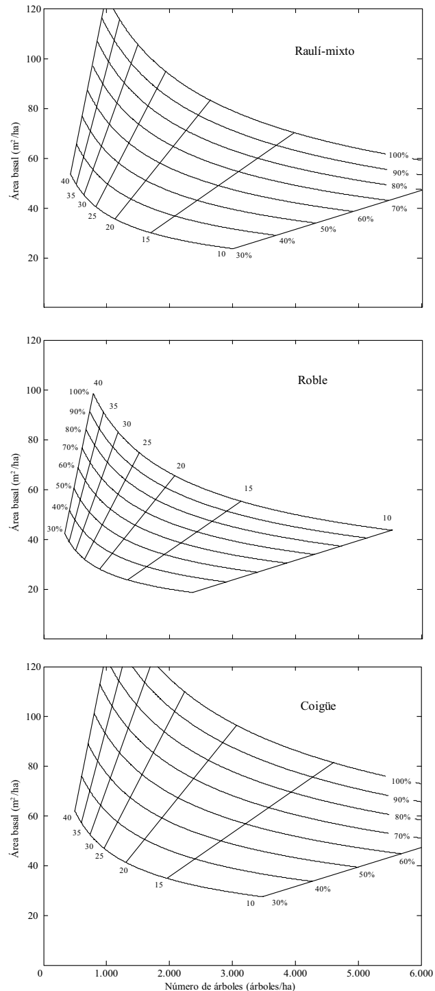
Figura 3. Diagramas de manejo de densidad para rodales de composición raulí mixto, roble y coigüe. Líneas indican diferentes diámetros cuadráticos (verticales) y niveles de capacidad de carga (horizontales).
