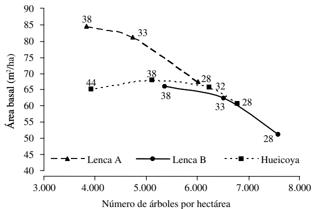
Figura 1. Curvas de densidad máxima a partir de parcelas testigo. Los números sobre las curvas representan la edad (años) del renoval.
