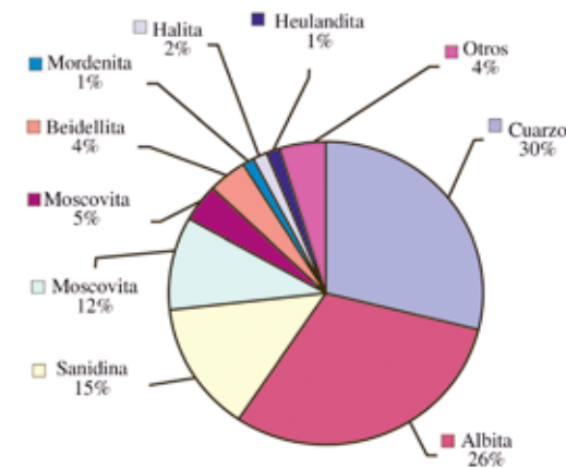
Figura 9. Promedio de los principales minerales encontrados en la Capa 3 (N = 8) mediante la técnica DRX y presentados en la Tabla 3.
