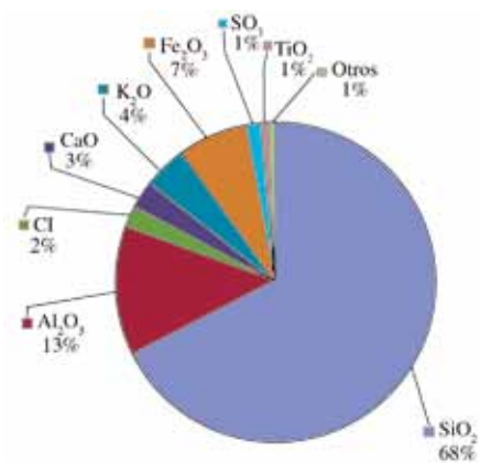
Figura 8. Promedio de los elementos químicos analizados en la Capa 3 (N = 13) utilizando la técnica EDXRF y presentados en la Tabla 2.
