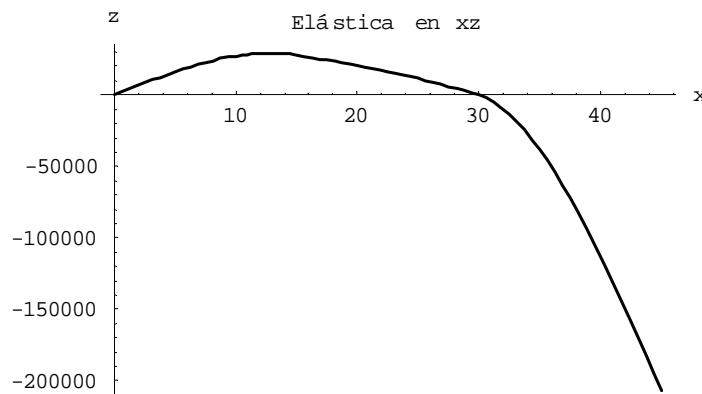
Fig. 5. Ejemplo de gráfica de la elástica en un caso de diseño. El valor de la flecha viene multiplicado por el valor de la rigidez el primer tramo del árbol, (EI)_1 .
