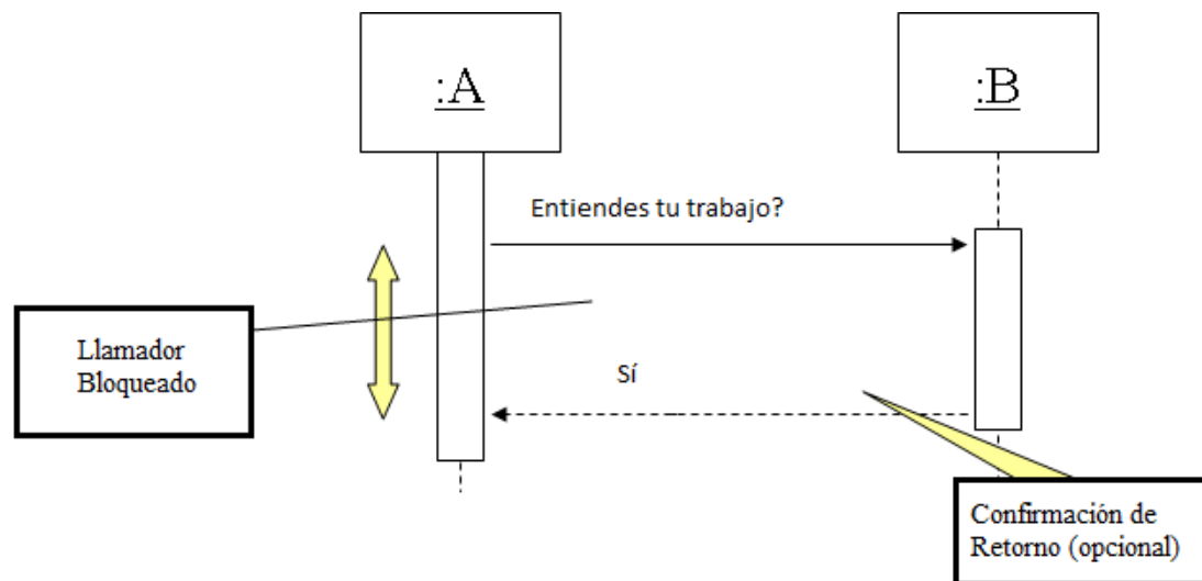
Fig. 2: Mensaje Síncrono y Flujo Continuo en Diagrama de Secuencias UML.
