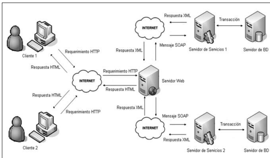
Figura 1. Diagrama de uso de servicios Web clásicos.
