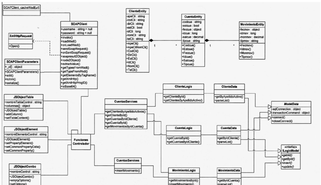
Figura 11. Diagrama de Clases del Prototipo.
