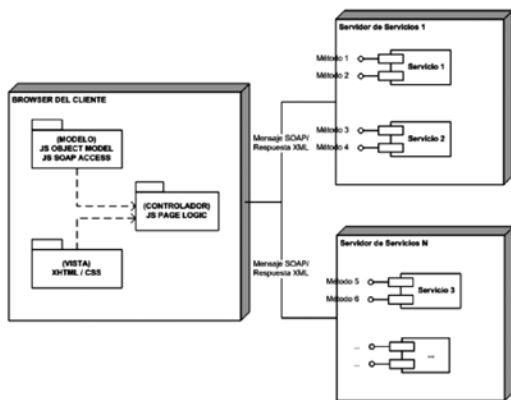
Figura 4. Diagnóstico de componentes del modelo propuesto.
