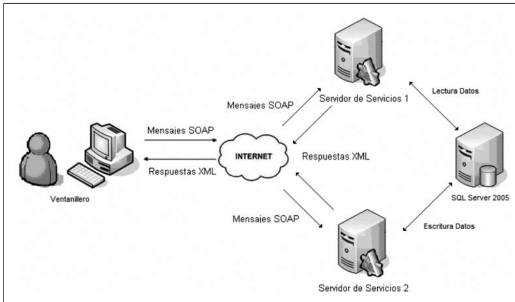
Figura 9. Diagrama de despliegue del prototipo.
