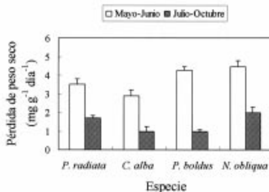
Fig. 2: Tasas diarias de descomposición de la hojarasca de cuatro especies arbóreas durante los primeros dos meses de incubación (mayo-junio) y durante los últimos cuatro meses (julio-octubre). Barras indican un error estándar. Para toda especie, las tasas diarias fueron significativamente mayores (prueba t de Student, P < 0,0001 ) durante los primeros dos meses que durante los últimos cuatro meses.
