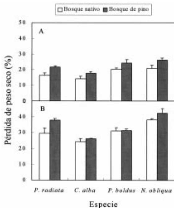
Fig. 1: Pérdida de peso seco de hojarasca, luego de (A) dos meses y (B) seis meses de incubación bajo bosque nativo y bajo un rodal de Pinus radiata . Barras indican un error estándar.
