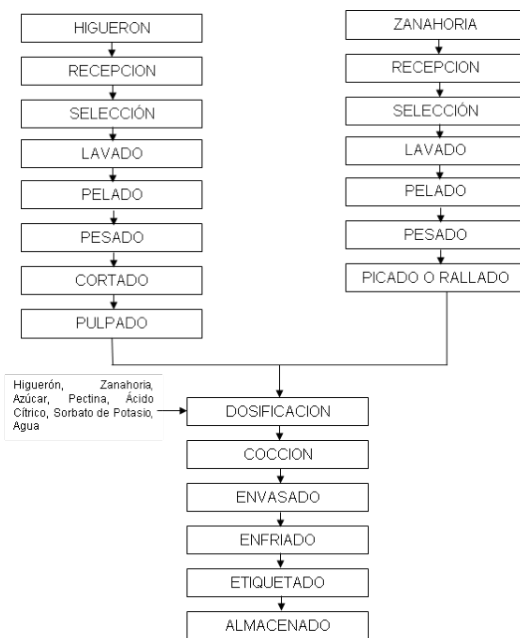
Diagrama de flujo de elaboración de mermelada de higuérón con zanahoria.
