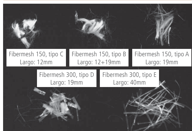
Ilustración 2. Todas las fibras poliméricas
