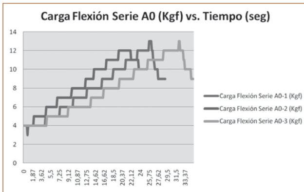
Ilustración 3.1. Gráfico Carga Flexión versus Tiempo, serie A0
