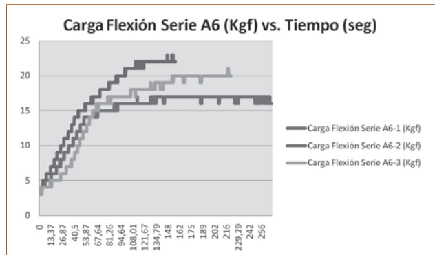
Ilustración 3.2. Gráfico Carga Flexión versus Tiempo, serie A6
